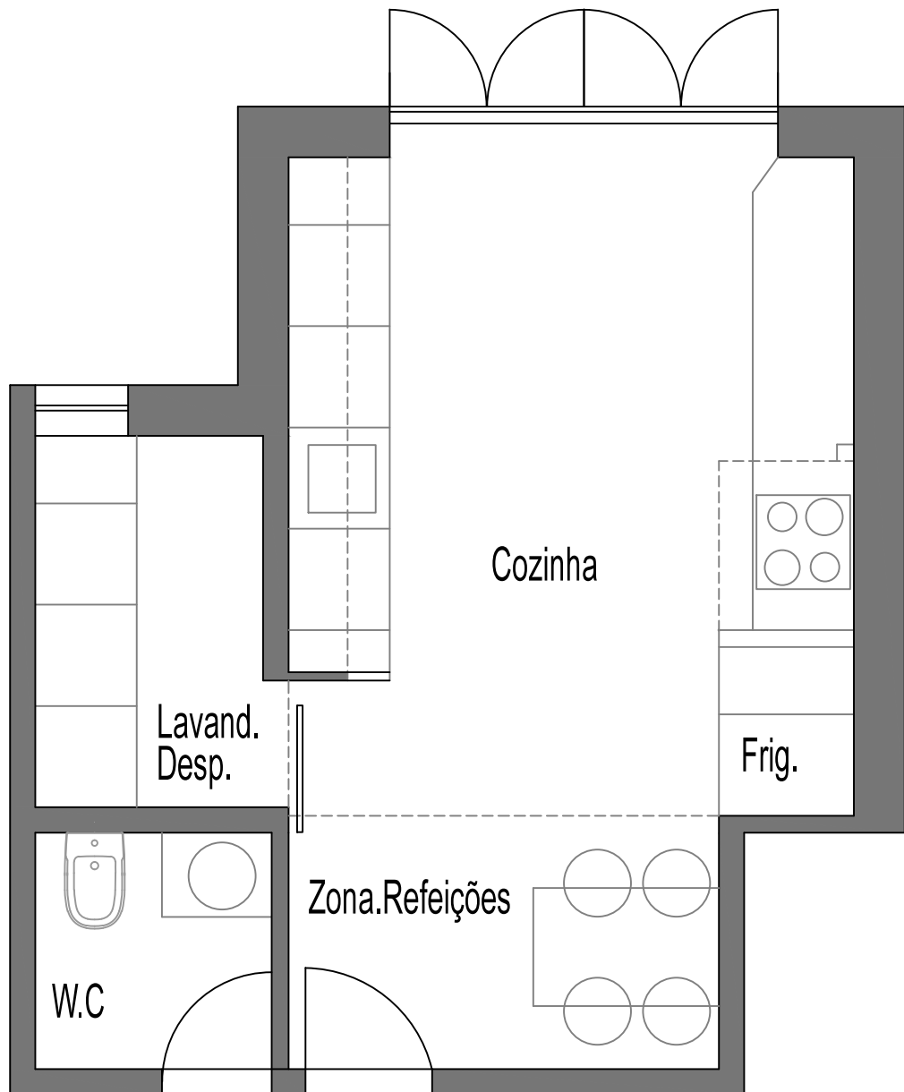
PLanta da proposta cozinha
